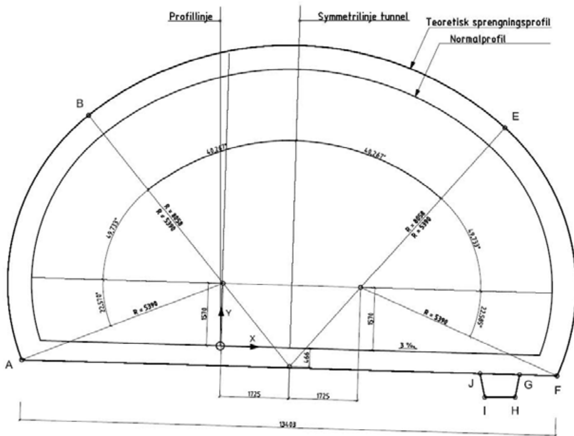
A TUNNELPROFIL - T12 S 125
